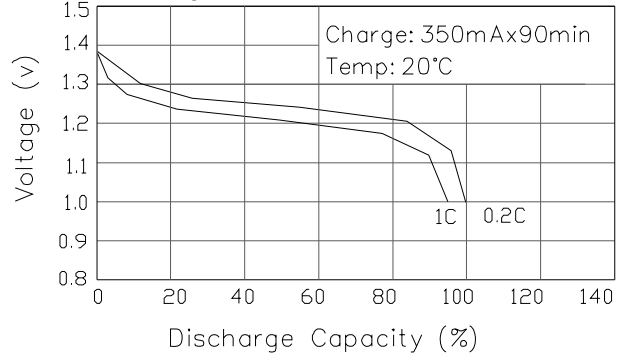
Discharge
