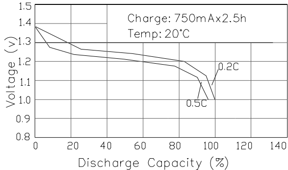
Discharge
